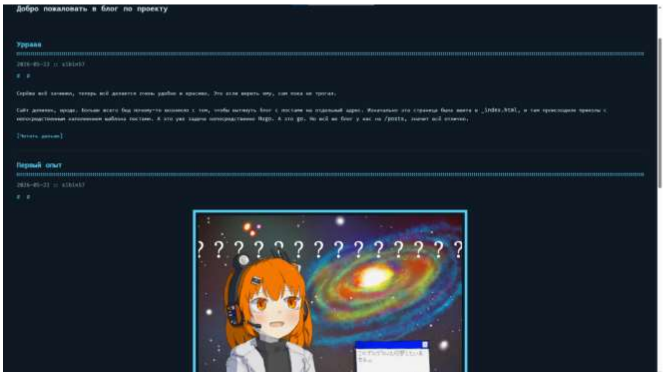
Рисунок 2. страница «Блог»
