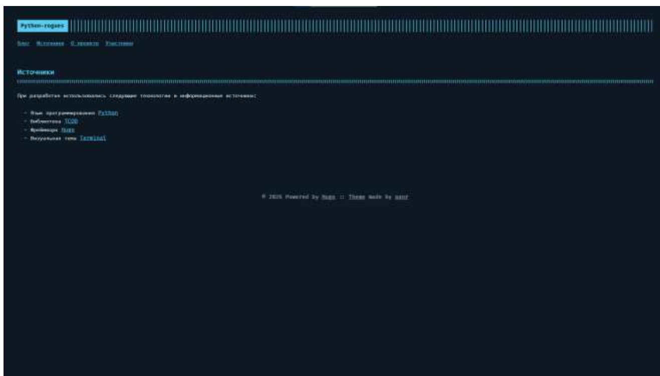
Рисунок 4. Страница «источники»
